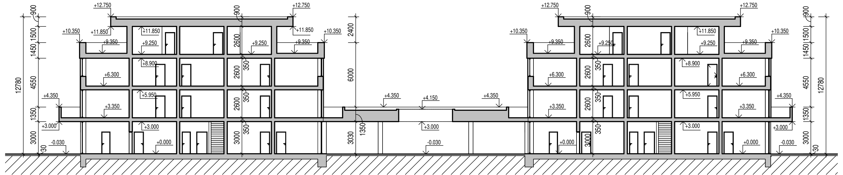
Rez A 1 : 200
